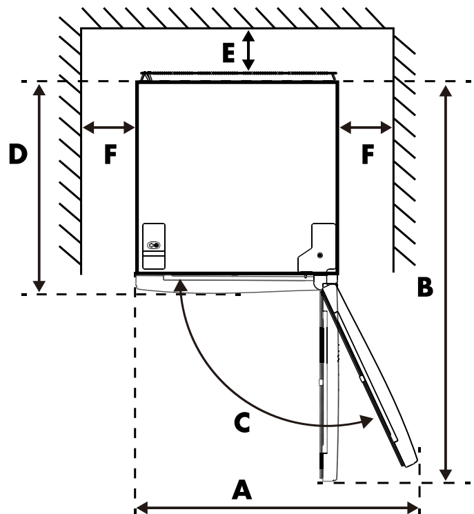
• Abbildung 2. Draufsicht
