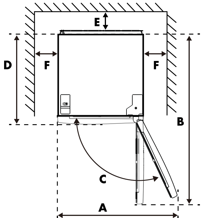
• Figuur 2. Bovenaanzicht
