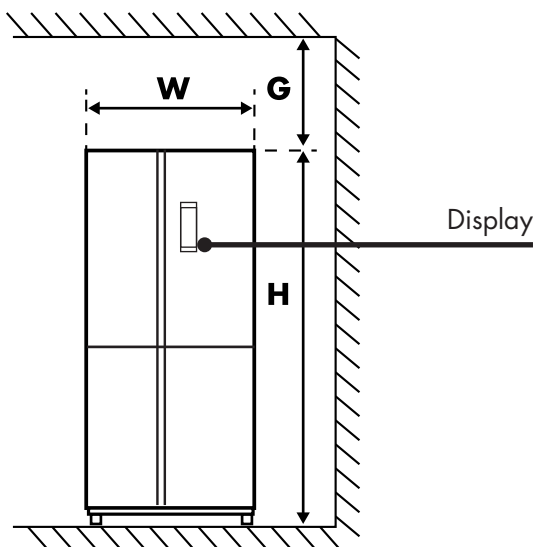
• Abbildung 1. Vorderansicht
