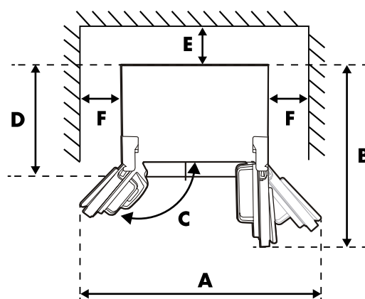
Figuur 2: Bovenaanzicht
