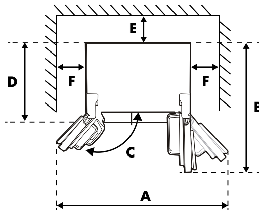
• Abbildung 2. Draufsicht
