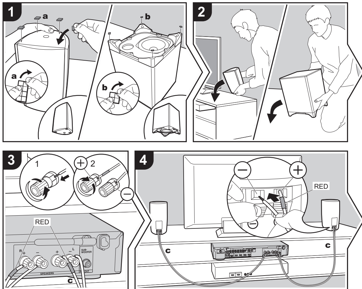
a Distanser för fronthögtalare, b Distanser för subwoofer, c Högtalarkabel
