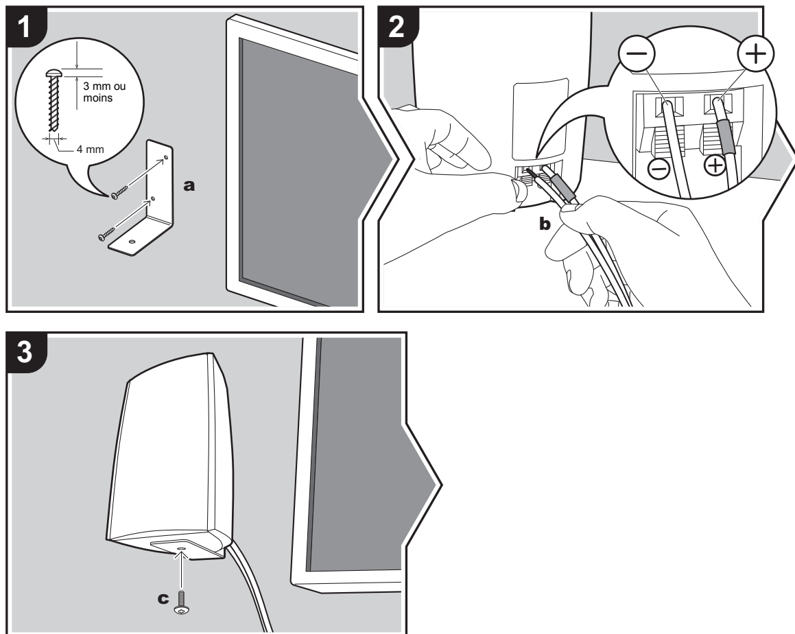
a Support du montage mural pour enceintes avant, b Câble d'enceinte, c Vis pour le support du montage mural (M5×10)
