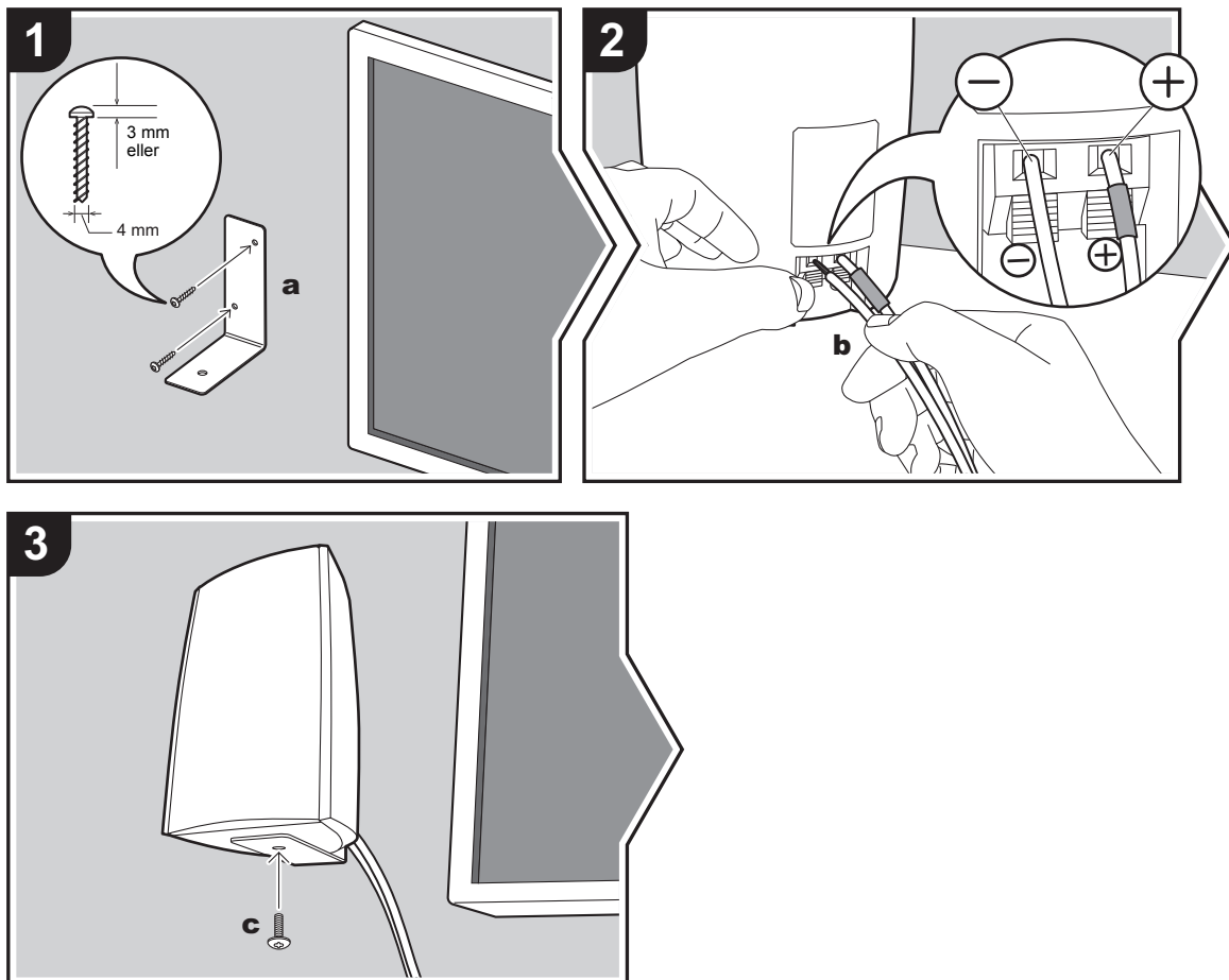
a Väggh monteringsfäste för fronthögtalare, b Högtalarkabel, c Skruv för väggh monteringsfäste (M5×10)
