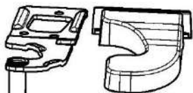
Cerniera superiore sinistra per la reversibilità dello sportello
